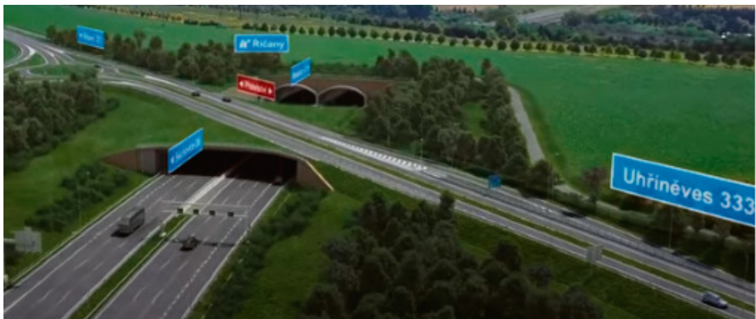
Dvoutubusový zahloubený tunel Na Vysoké měří 394 metrů.
