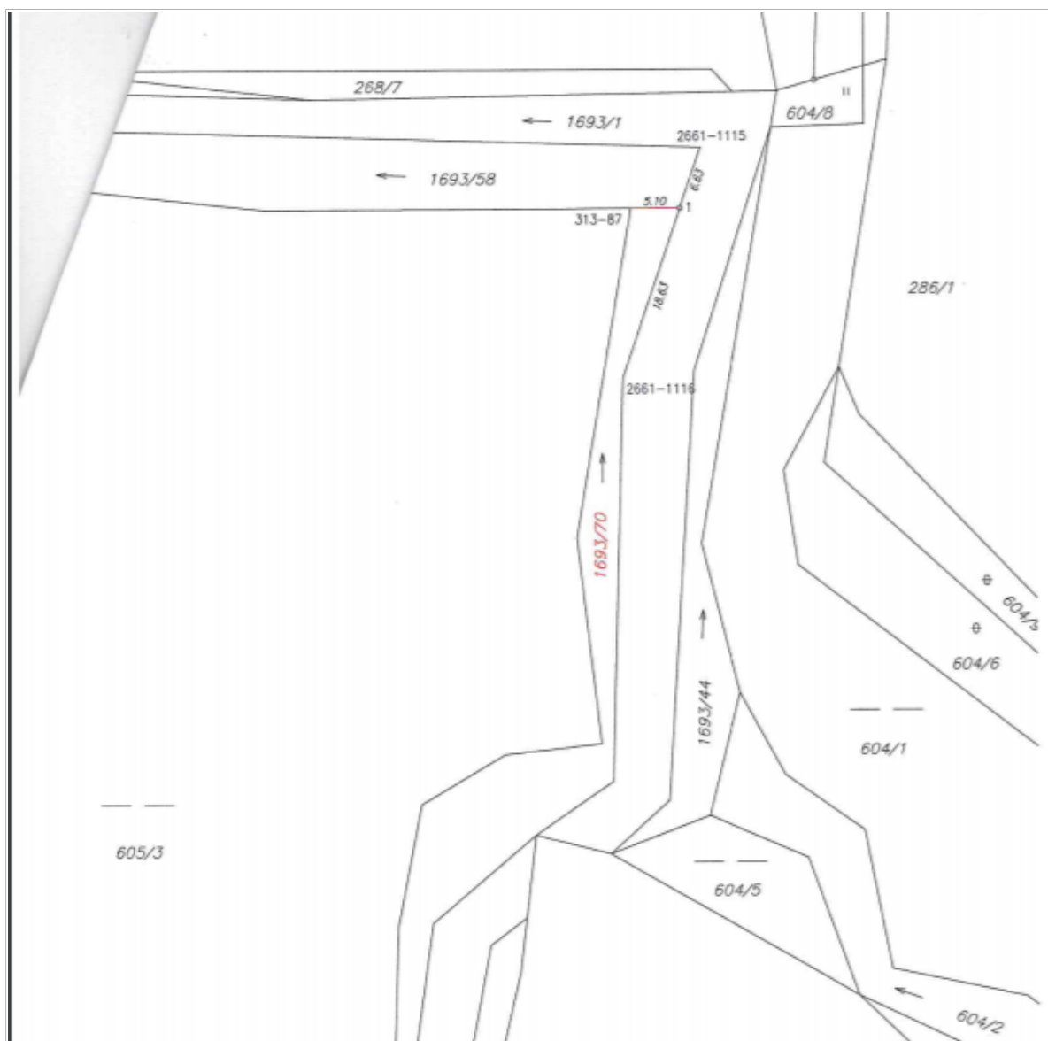
Geometrický plán – pozemek pod rybníkem Rozpakov
