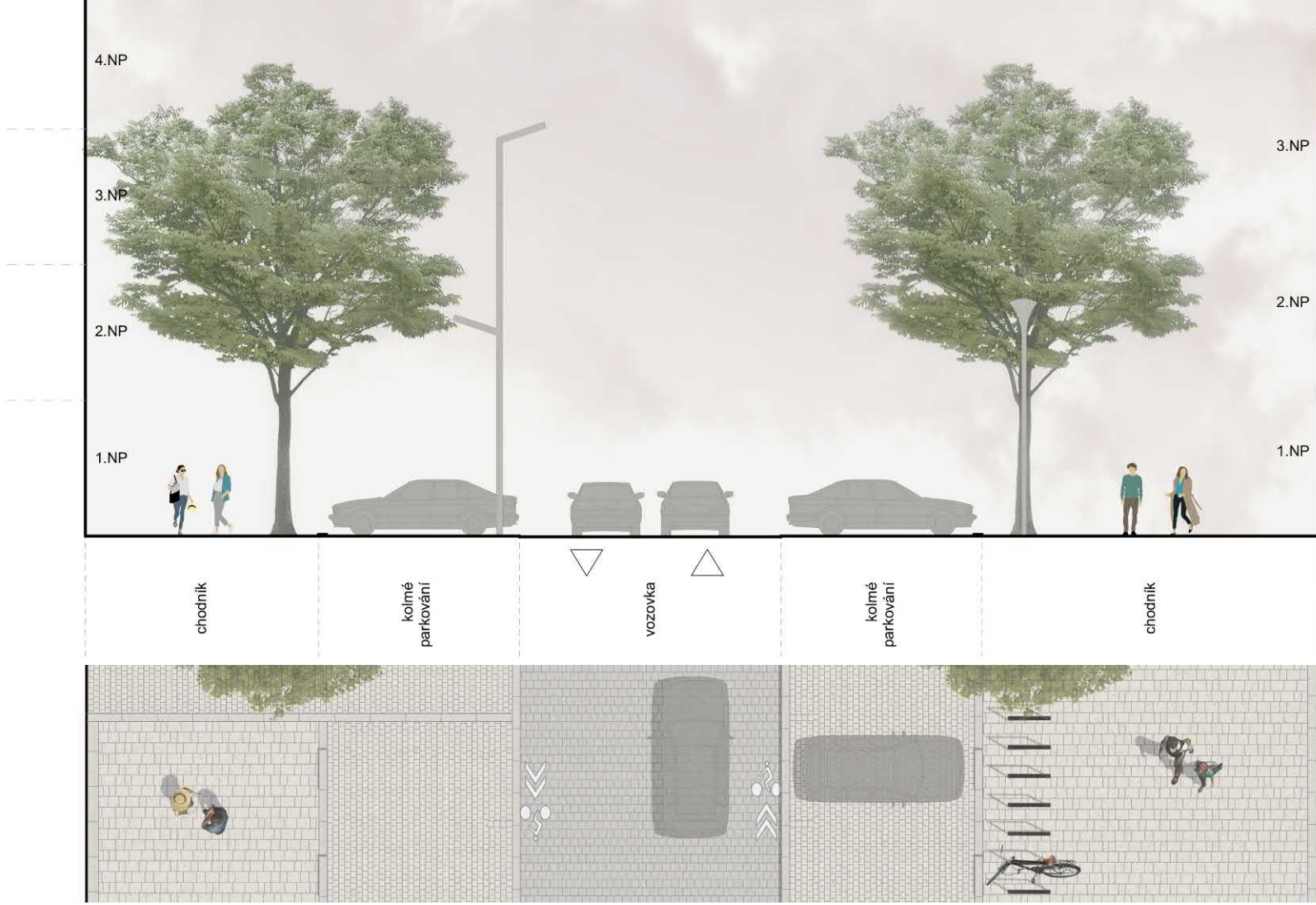
▲ ULIČNÍ PROFIL NA JIŽNÍ STRANĚ NÁMĚSTÍ 1:150
