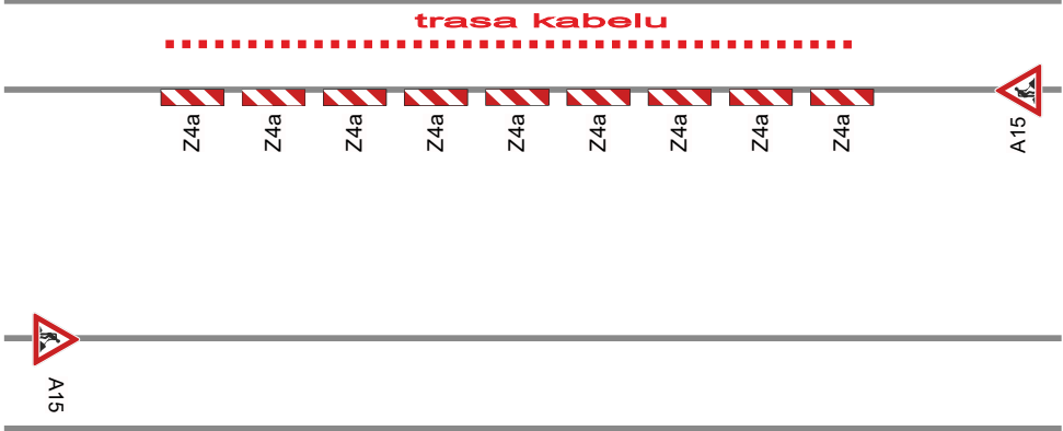
schéma SDZ
